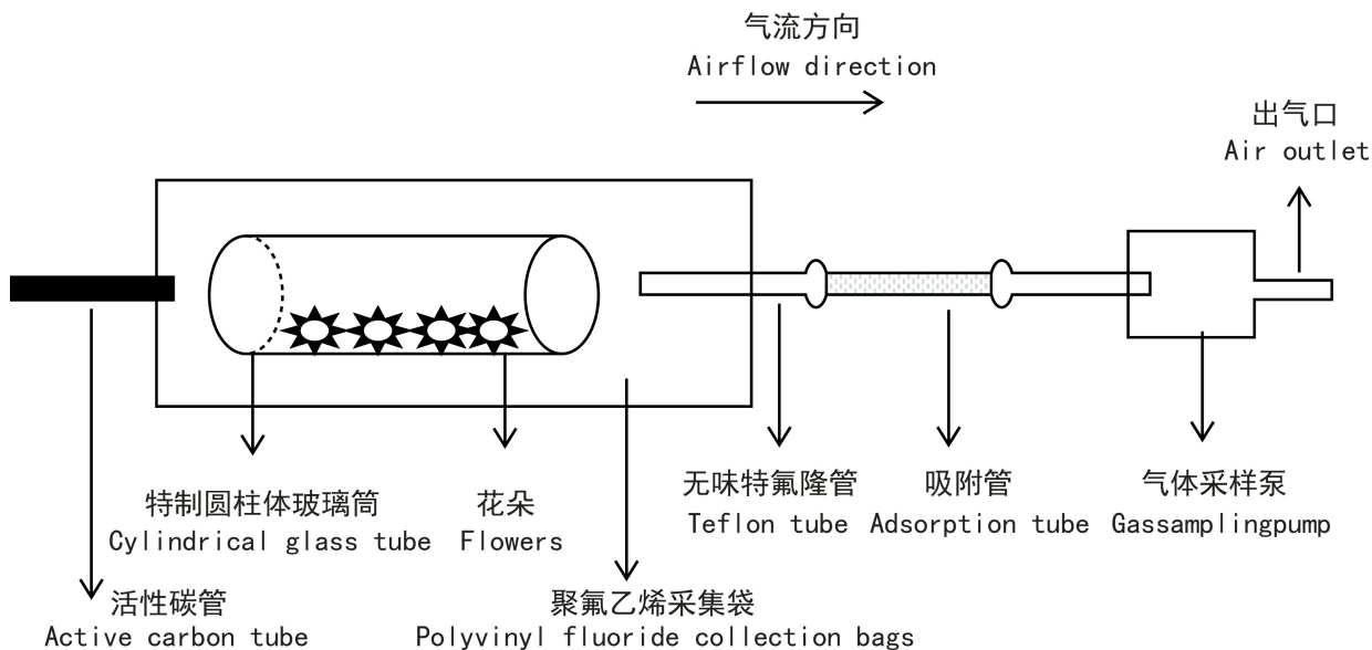
图 1 花气味物质收集装置图
