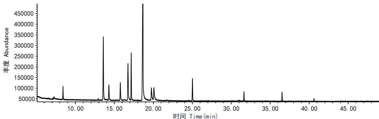
图 2 洗脱液 GC-MS 分析总离子流程图
